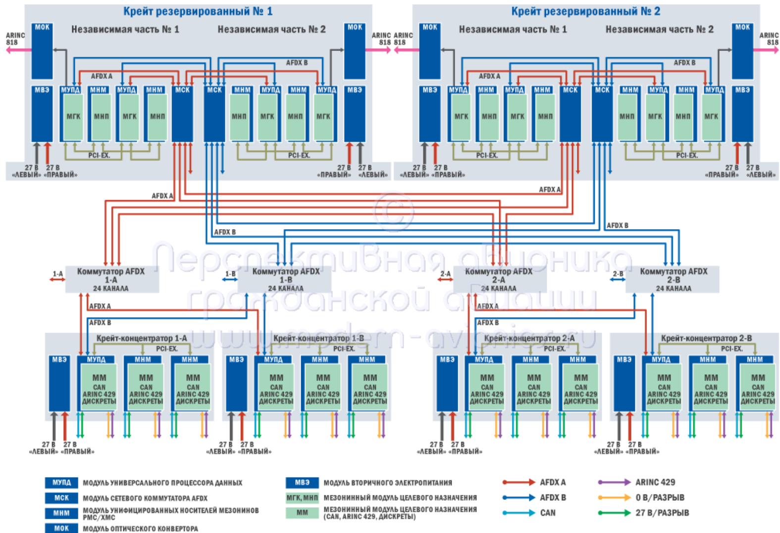
Рисунок 24 – Структурная схема платформы ИМА [87]
