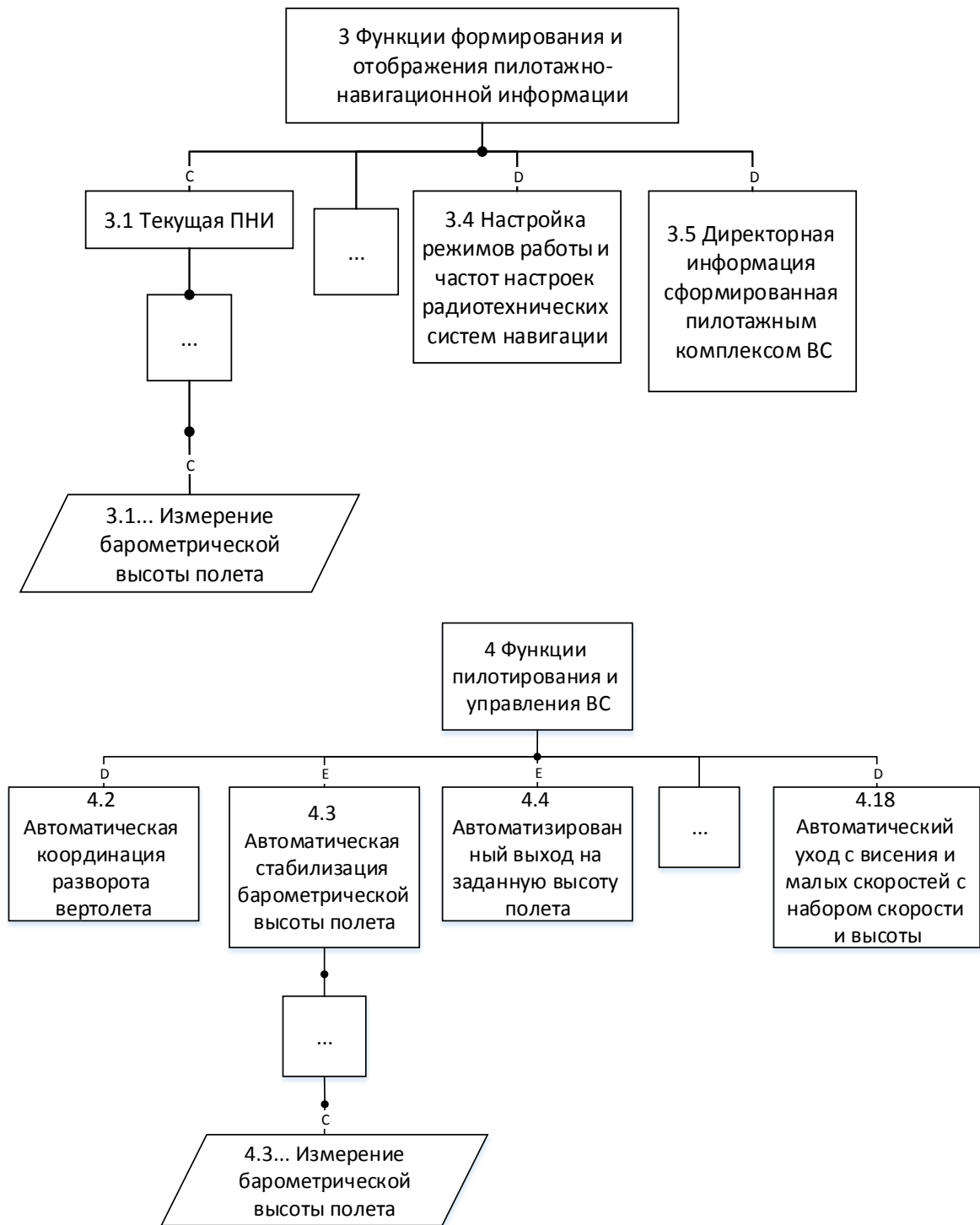
Рисунок 33 – Фрагменты структуры функций КБО
