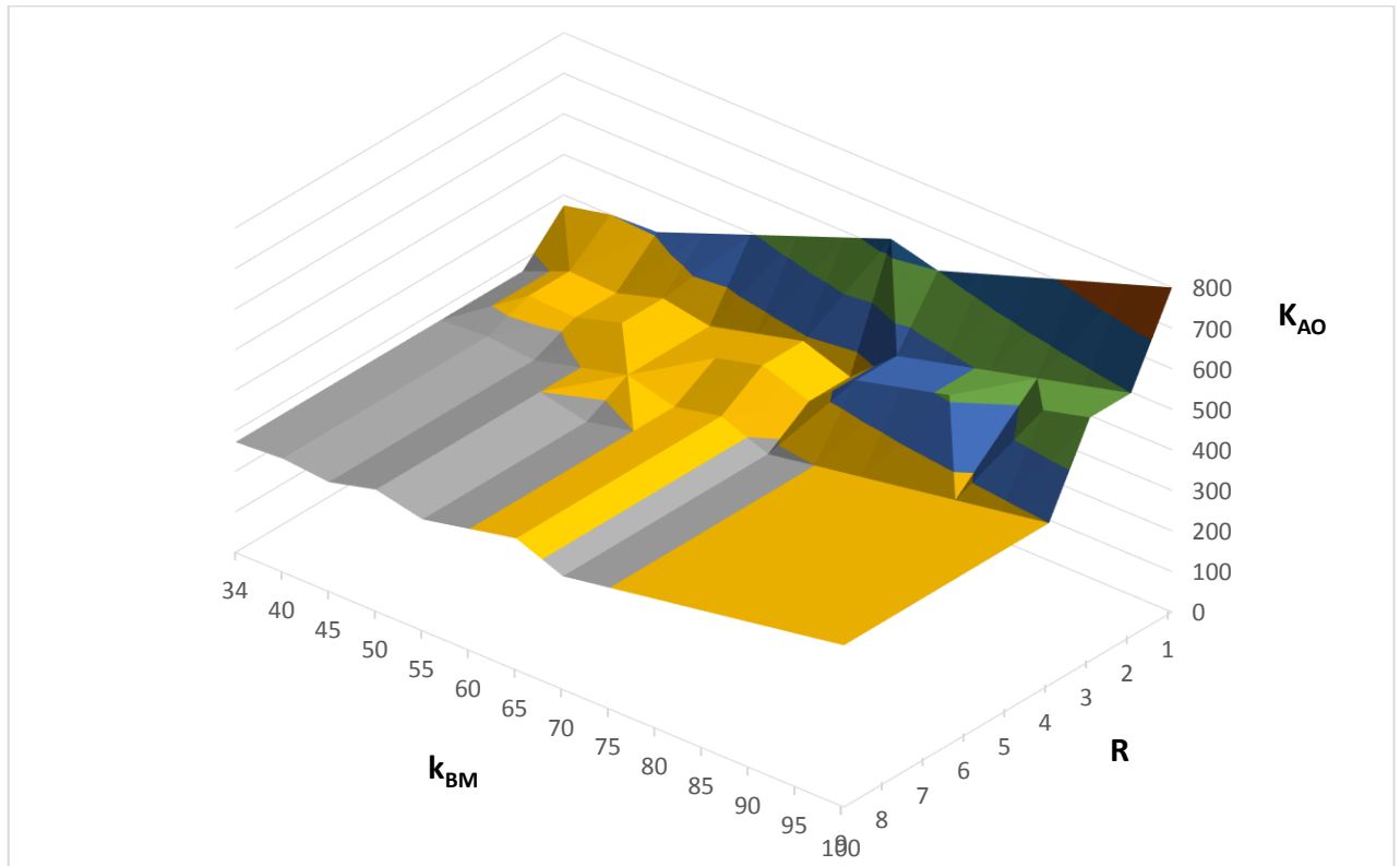
Рисунок 30 – Поверхность значений КВР АО
