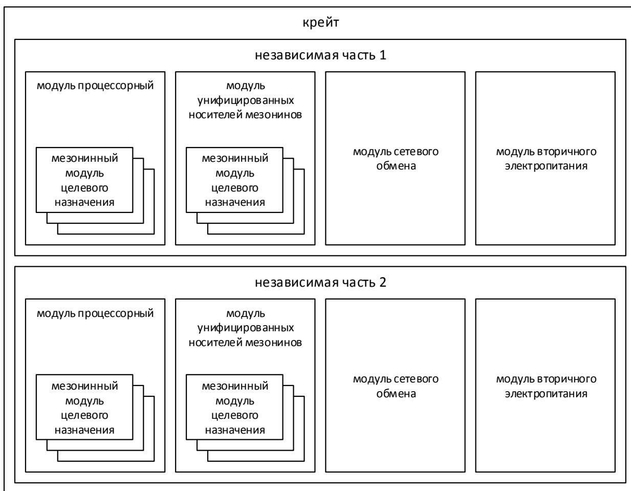
Рисунок 13 - Типовая структура крейта
