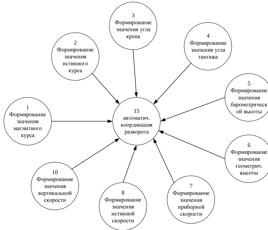
Рисунок Б.1 – Первичная структура функций, подграф 1
