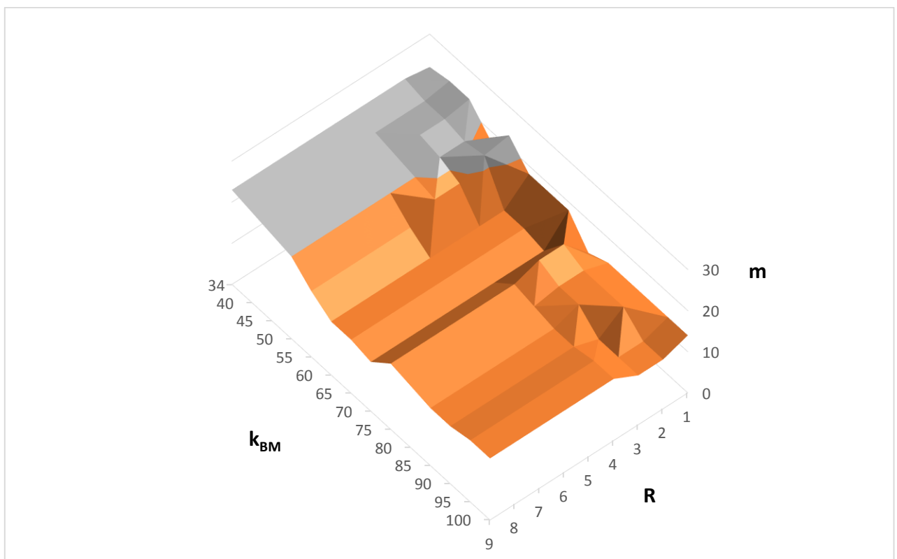
Рисунок 31 – Поверхность значений количества связей
