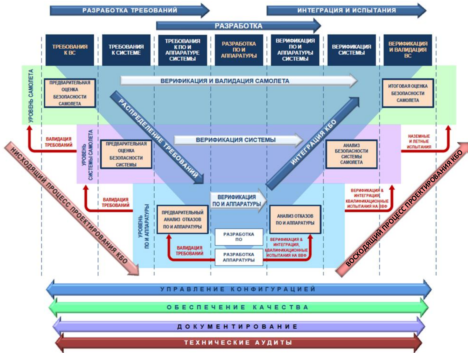
Рисунок 15 – Модель процесса проектирования авионики [4, 5]
