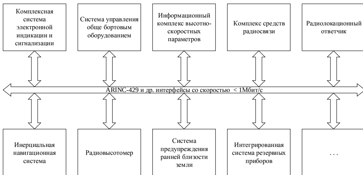
Рисунок 5 - Типовая схема КБО второго типа
