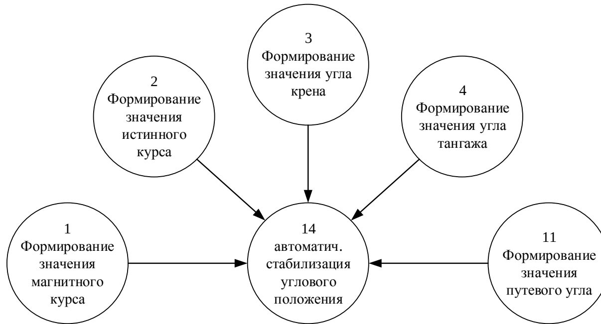
Рисунок Б.2 – Первичная структура функций, подграф 2
