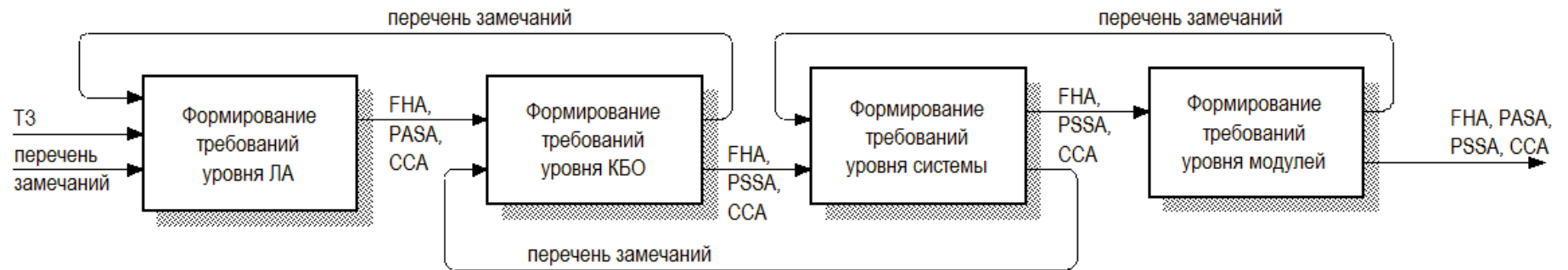
Рисунок 18 – Модель этапа формирования требований процесса оценки безопасности
