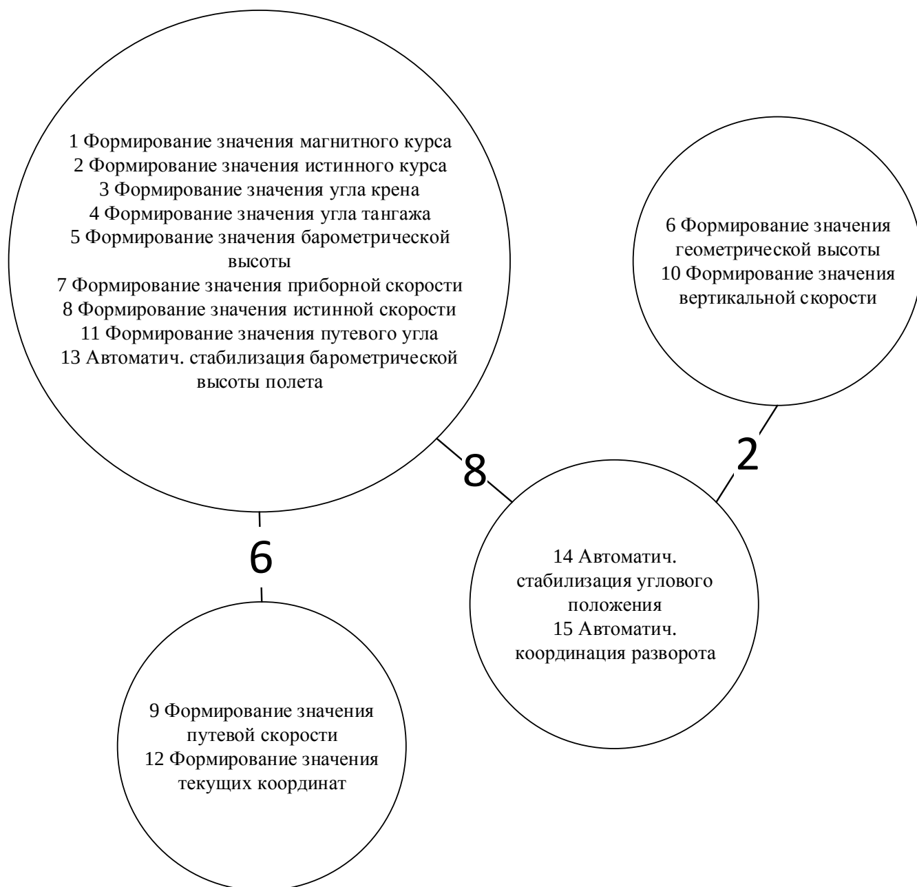
Рисунок 32 – Граф конечной структуры функций
