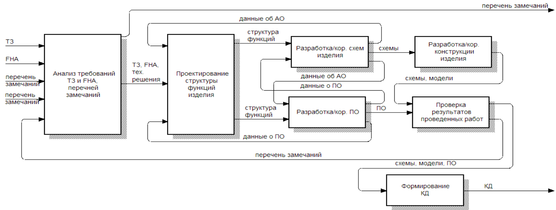
Рисунок 21 – Модель эскизного этапа процесса проектирования КБО ИМА, включающая процессы оценки безопасности и проектирования структуры функций
