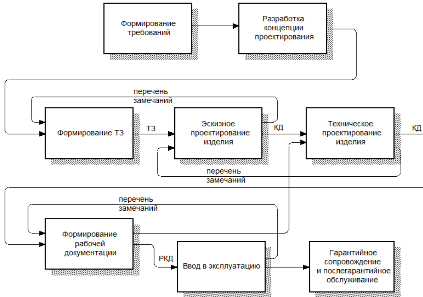
Рисунок 16 – Модель процесса проектирования
