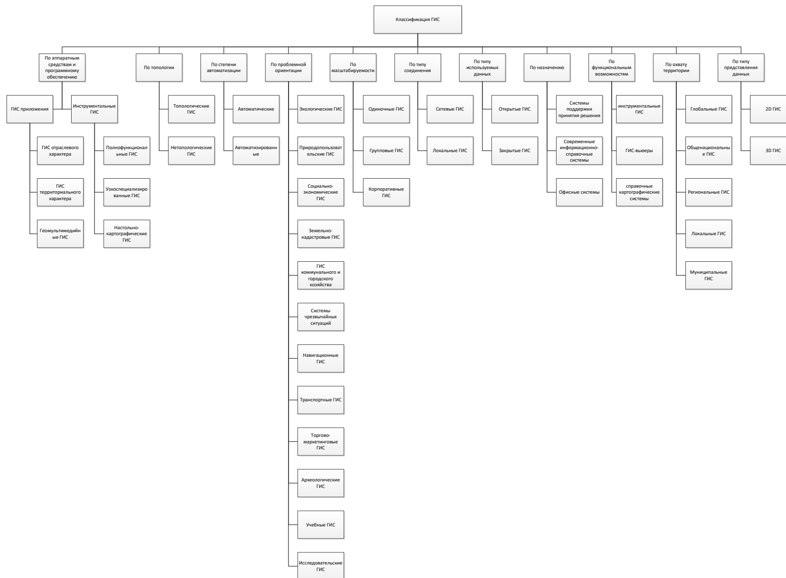
Рисунок 1.1. Классификация ГИС
